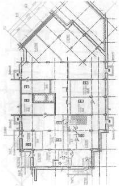
План Объекта долевого строительства-2 (секция № 1, цокольный этаж)
